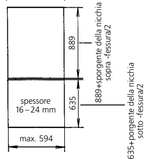
panello della porta EU
